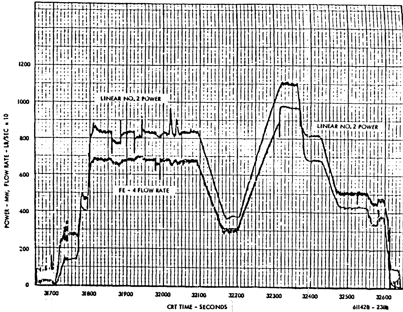
NRX/EST EP-III, Run 2 Profile (Sheet 2) - 3400°R Mapping
